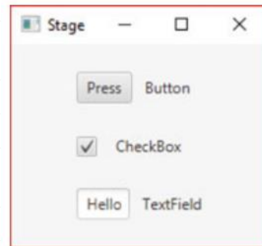
JavaFX
