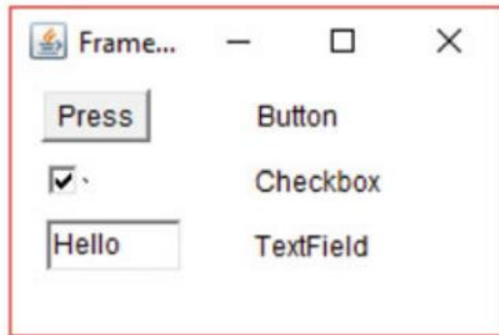
AWT
